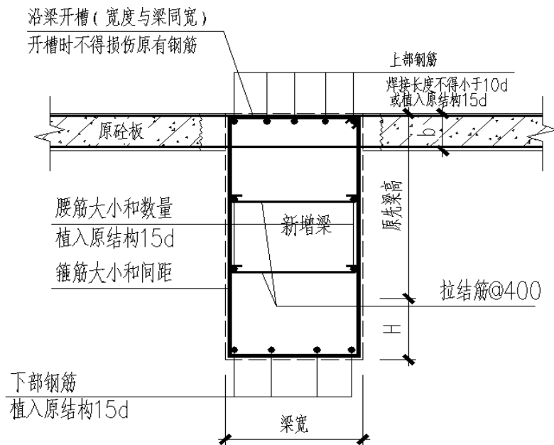
15-1 板下新增砼梁（二）
