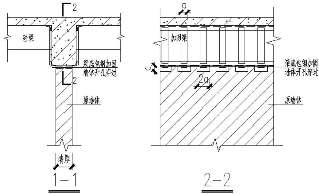
16-4 梁底粘钢（碳布）时，加固处理方法
