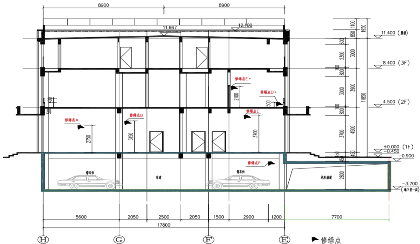
图21-1 室内垂直运输计算示例 (1: 100)
