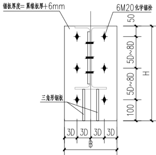
钢梁锚板
