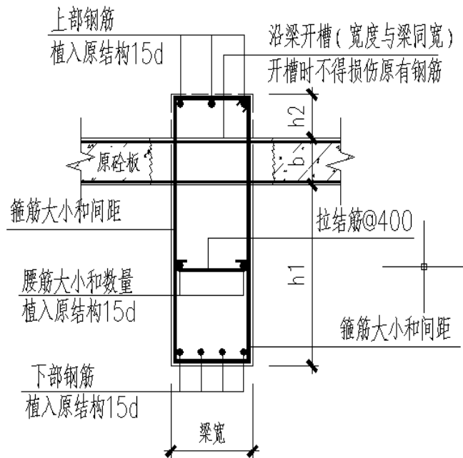
15-1 板下新增砼梁 (三)
