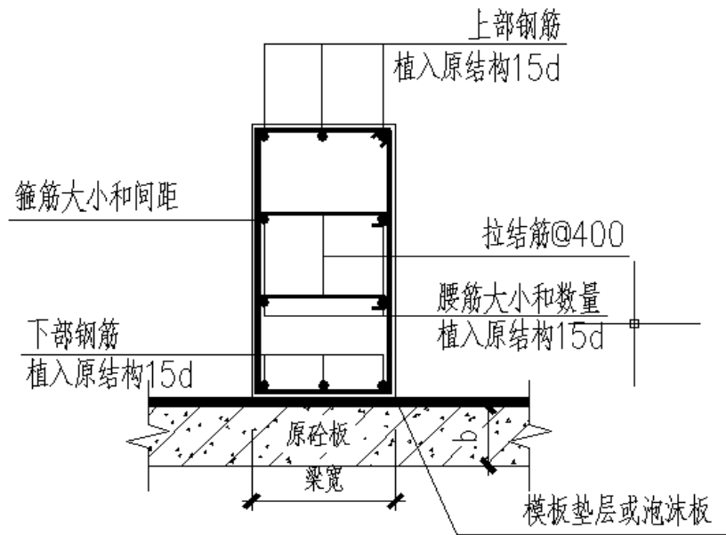
15-1 板下新增砼梁 (四)
