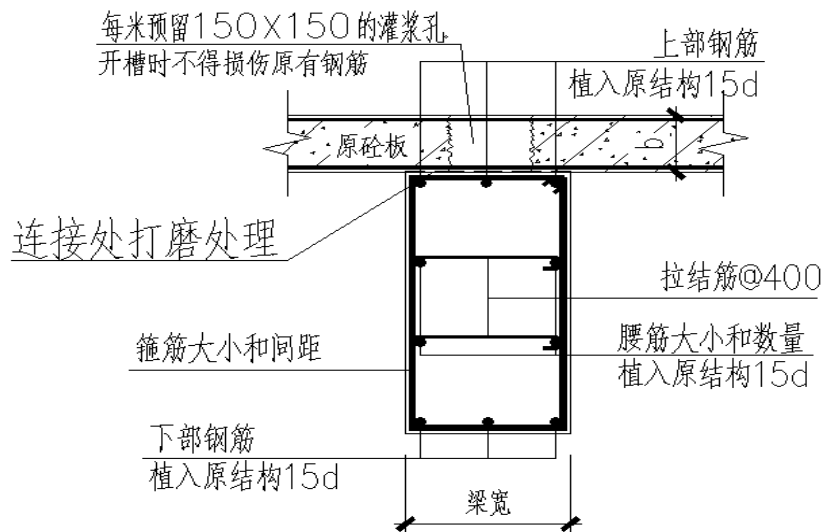
15-1 板下新增砼梁（一）
