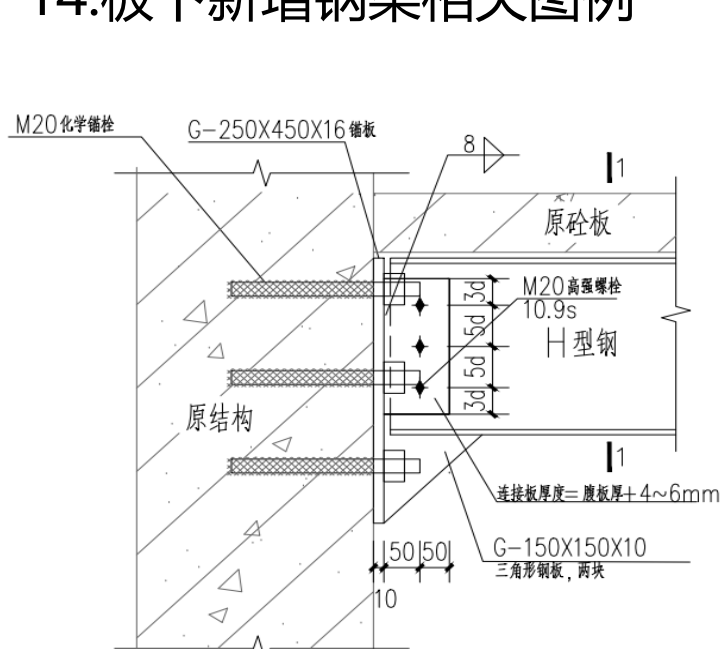
板下新增钢梁
