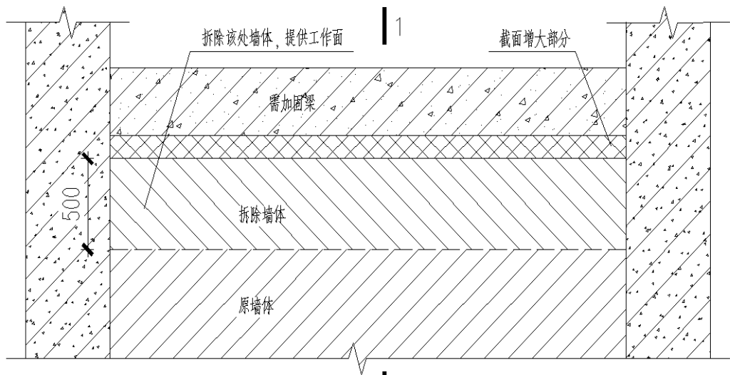
加固梁遇墙处理示意图
