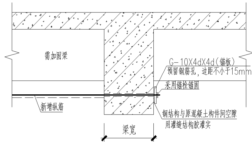
植筋后锚固示意图
